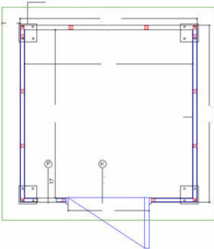
SİSTEM ODASI DEMİR KONTRÜKSİYON PLANI
