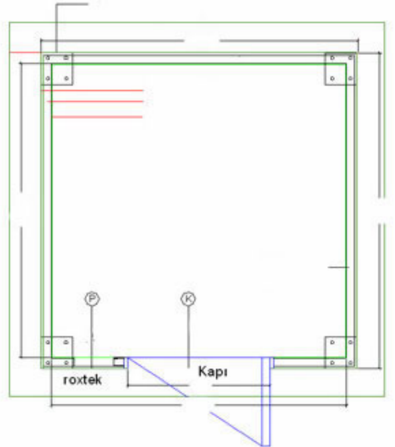
SİSTEM ODASI KAPLAMA VE KONTRÜKSİYON PLANI
